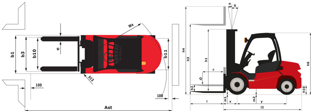
MI 50 LD ST5 - Disegno quotato
